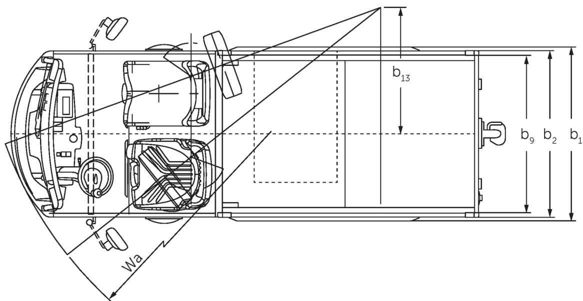
Typový list, EZW, technický výkres
