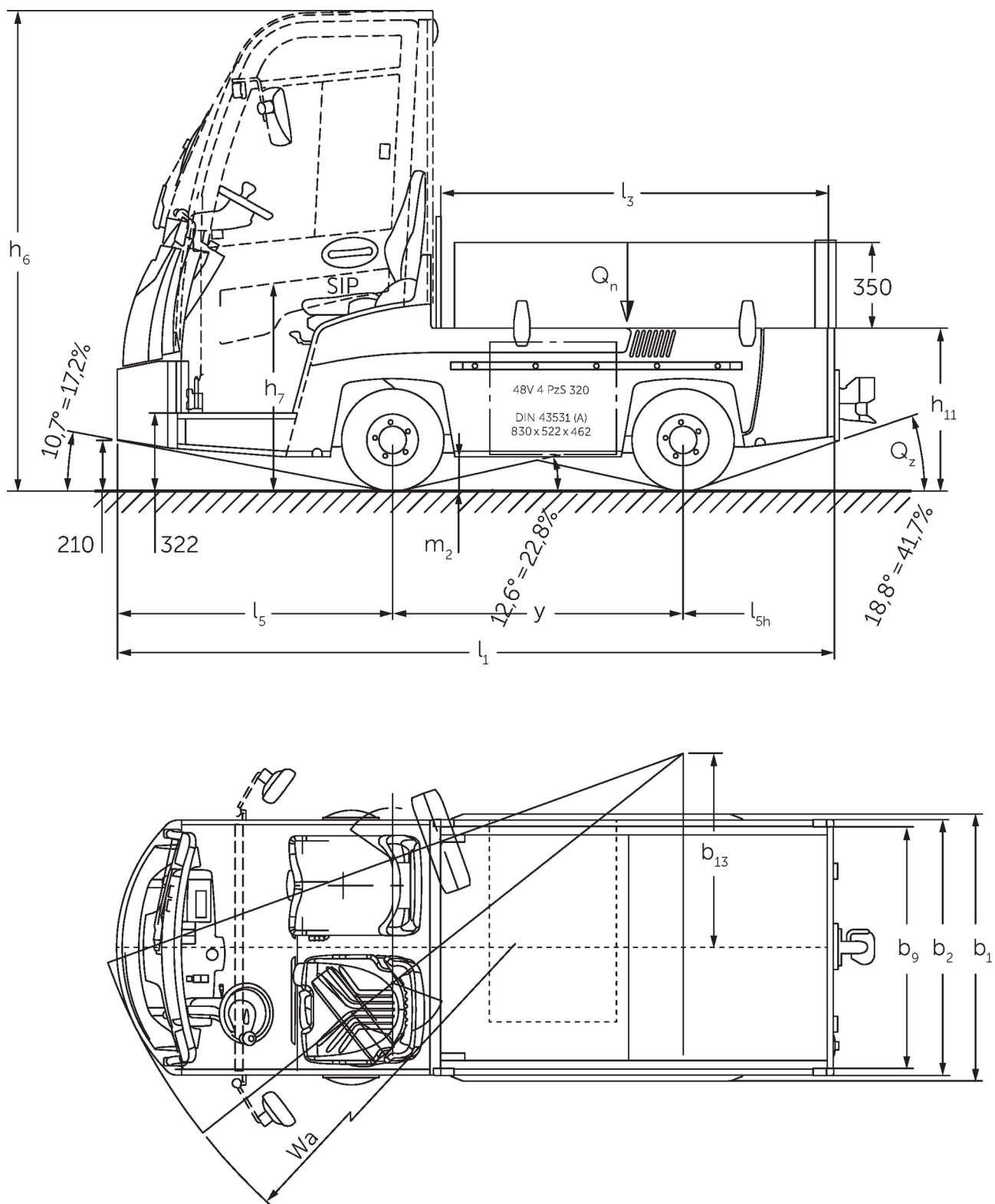
Технические данные, EZW, технический чертеж
