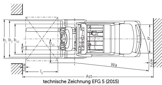
technische Zeichnung EFG 5 (2015)
