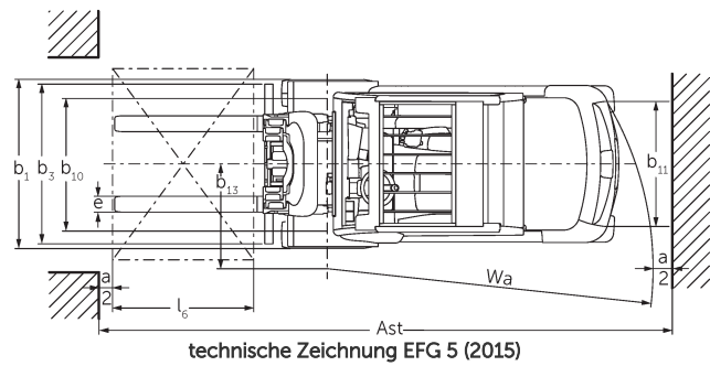
technische Zeichnung EFG 5 (2015)
