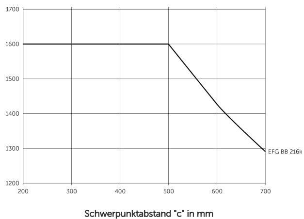
Tragfähigkeit (kg)
