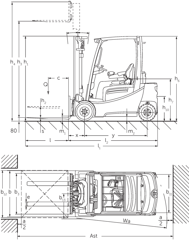
EFG 3 technische Zeichnung 2016
