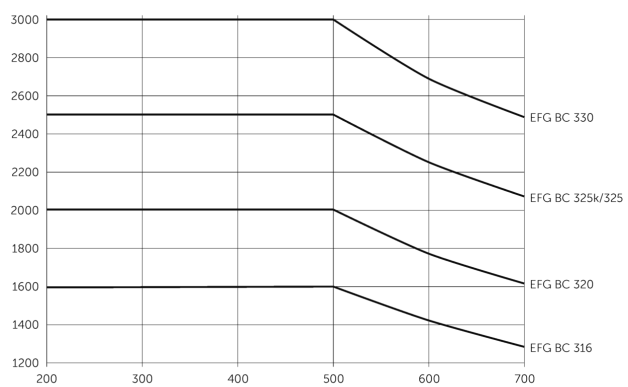
Tragfähigkeit (kg)
