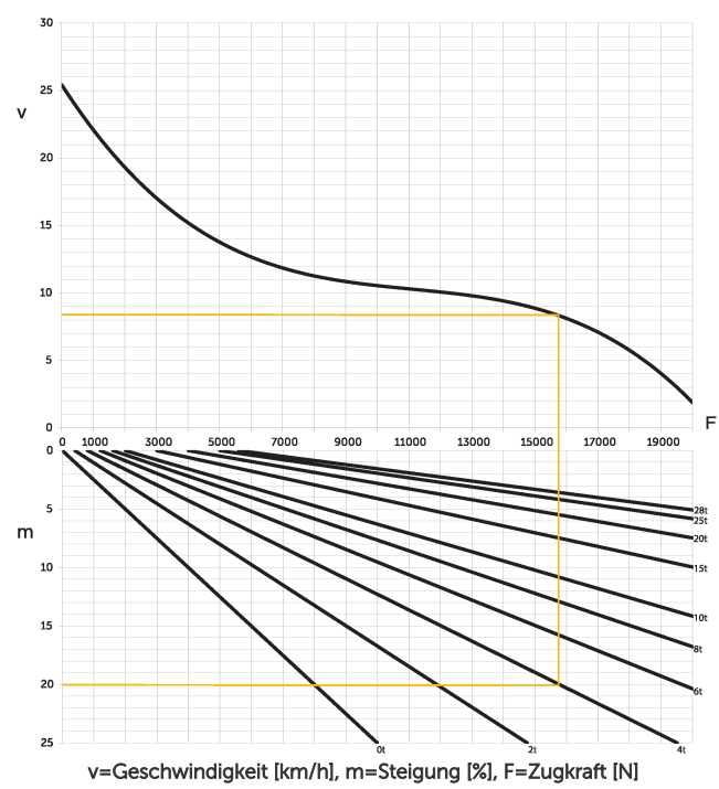
Zugfähigkeit
