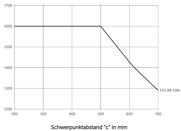
Tragfähigkeit (kg)
