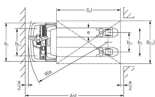
Linjeritningar EJE
