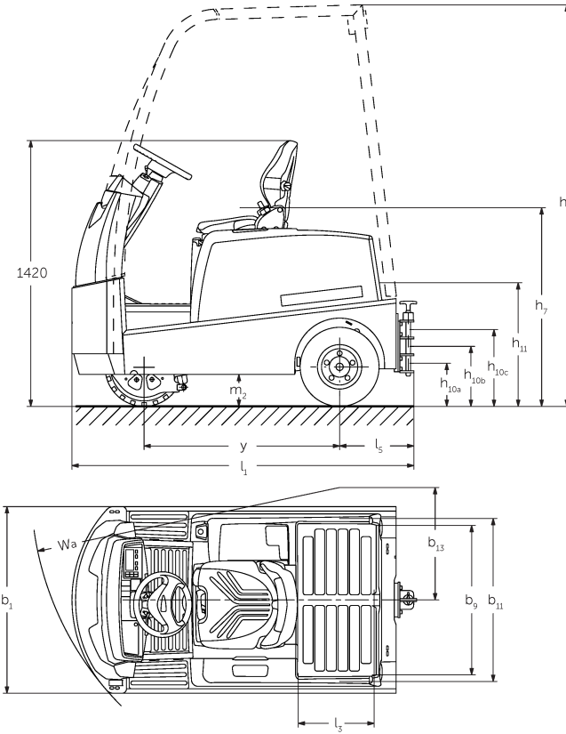
EZS 580, teknisk ritning, typblad
