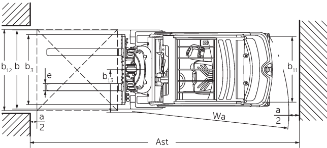
EFG 3 teknisk ritning 2016
