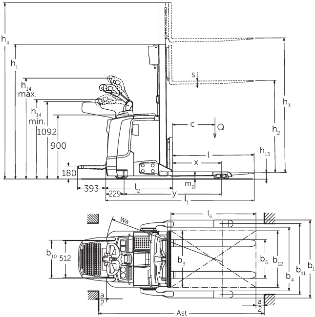
Måttitning ERC 2b
