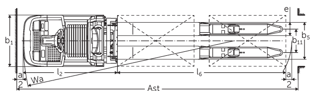
ECD 320 NOC 2016 teknisk ritning
