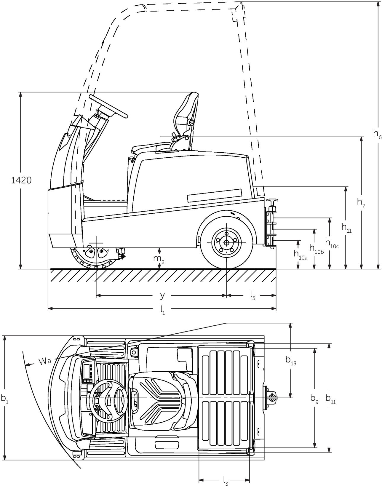
EZS 580, technische Zeichnung, Typenblatt Zugfähigkeit
