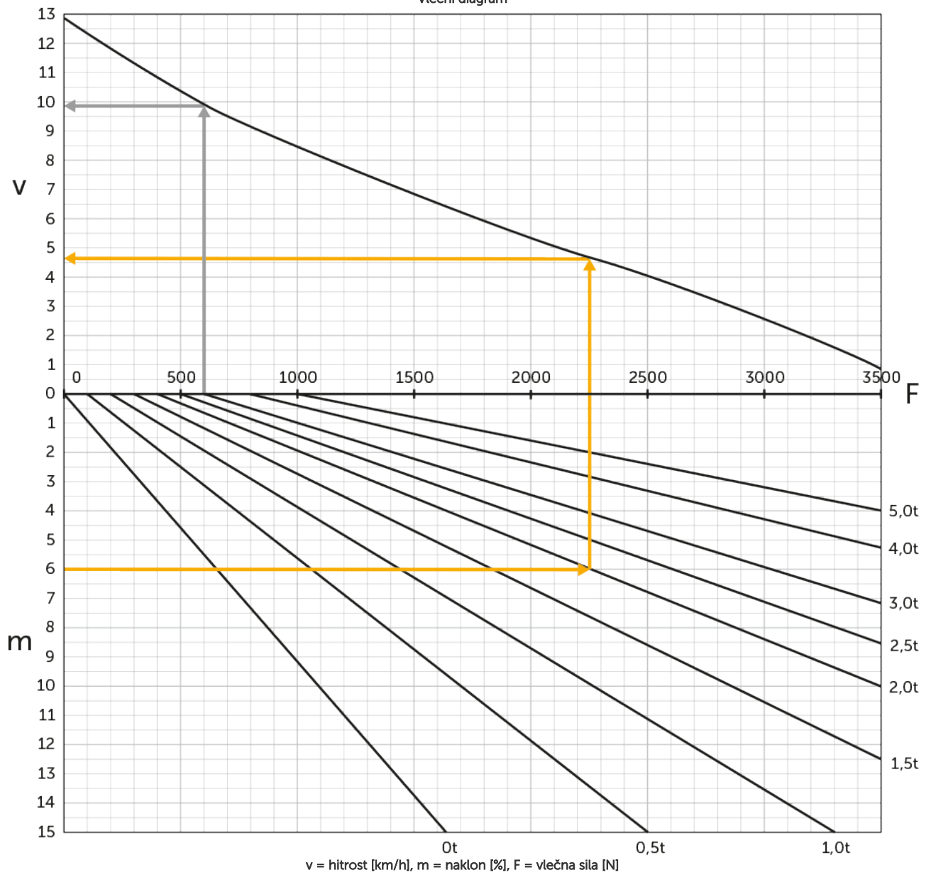
Vlečni diagram
