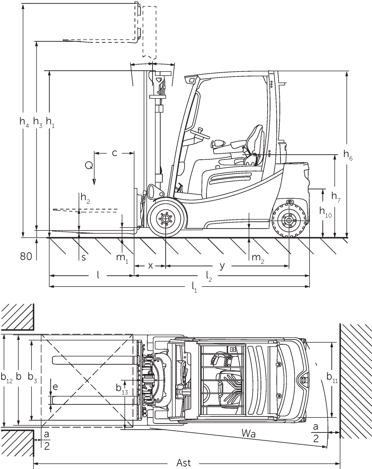
EFG 3 rysunek techniczny 2016
