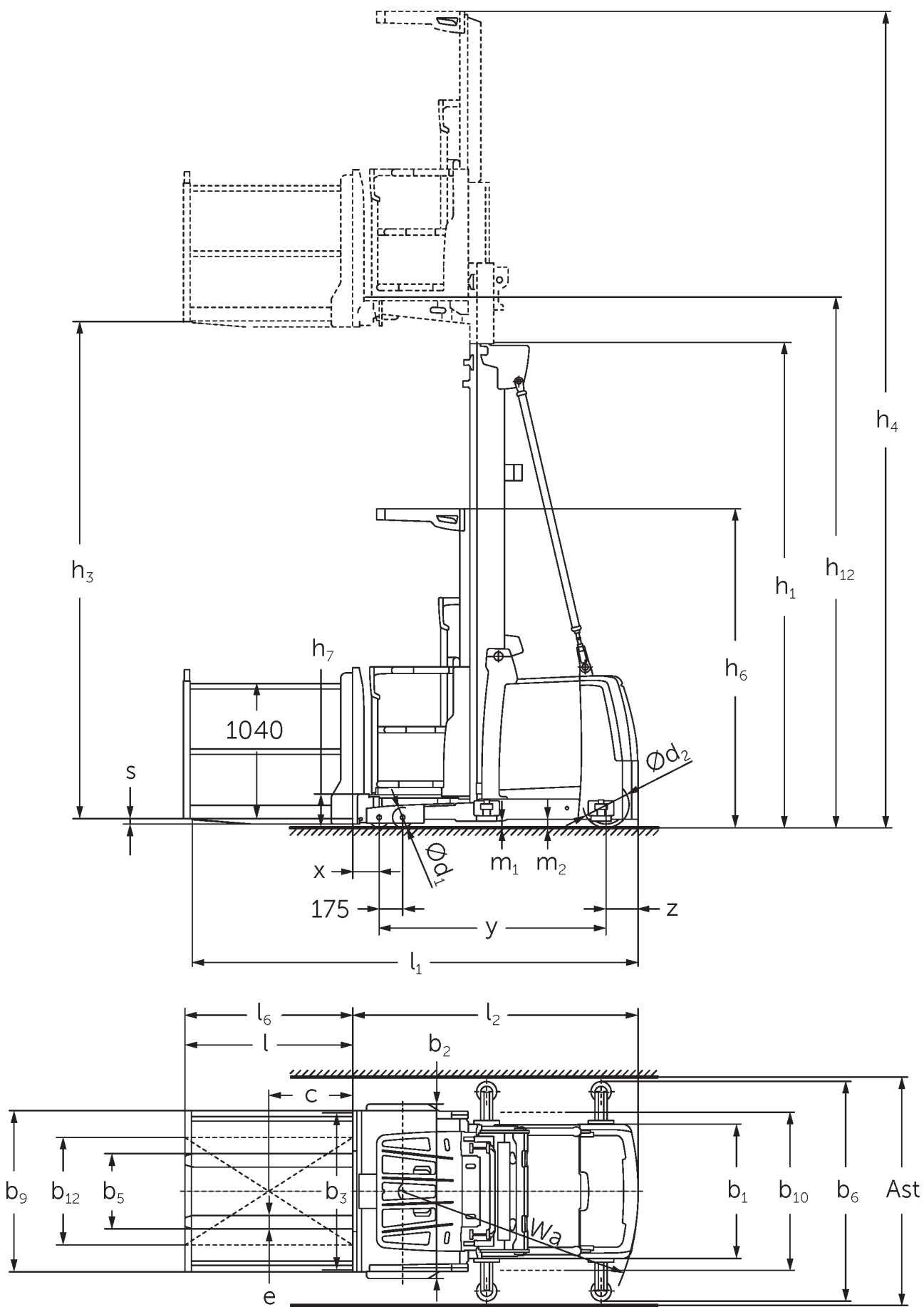
Disegno tecnico della versione EKS 3/4 L
