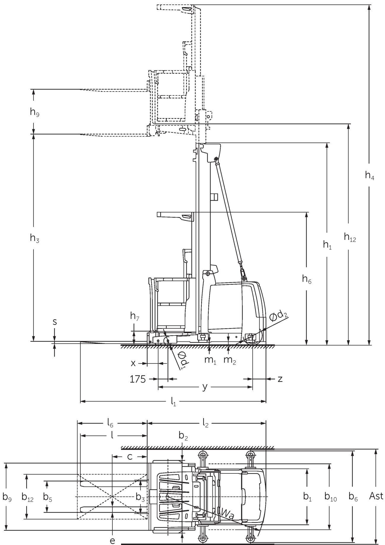
Dibujo técnico de la versión EKS 3/4 Z
