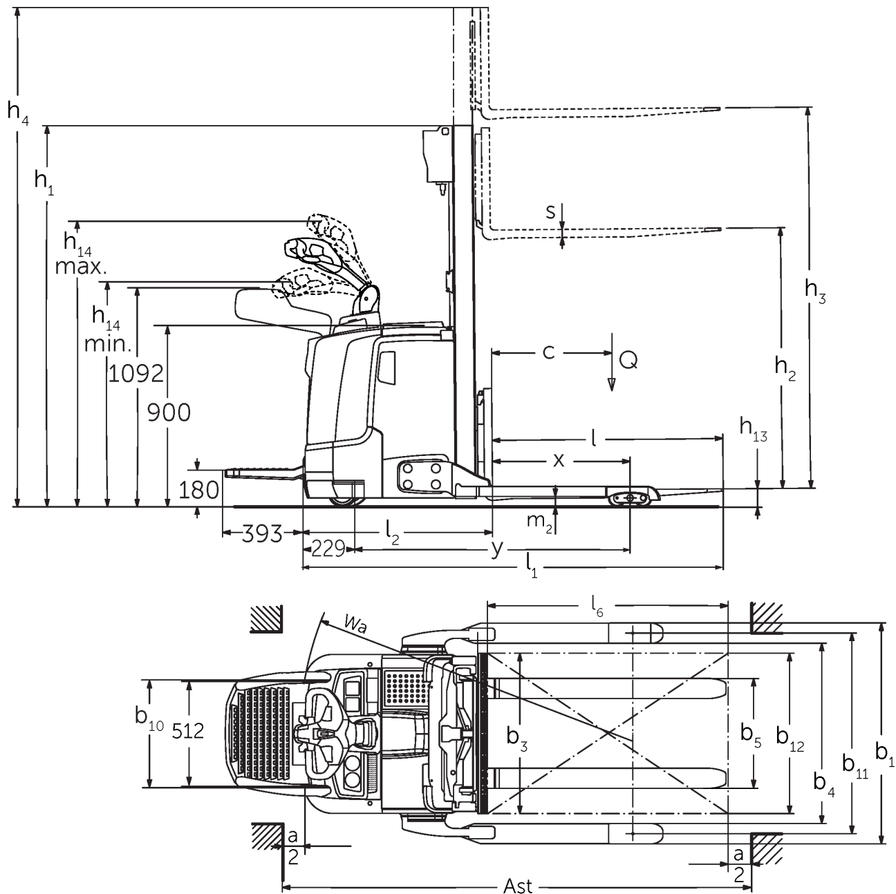
Måttitning ERC 2b
