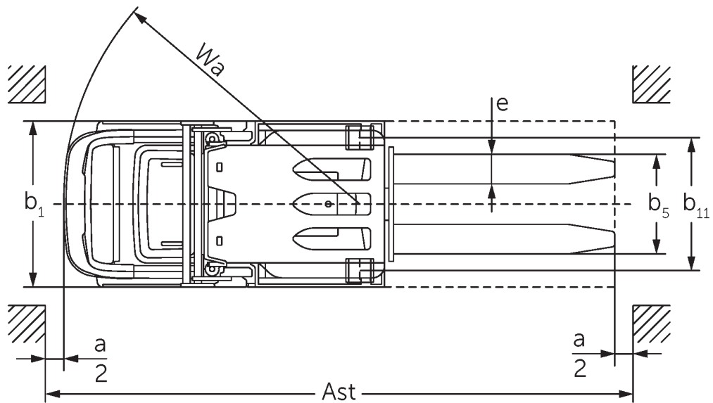
Afbeelding van de EKS 110 Z 280 ZZ
