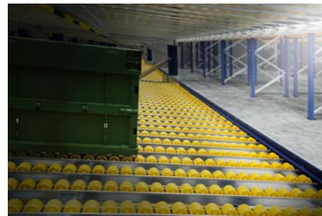
Spádový valčekový systém
