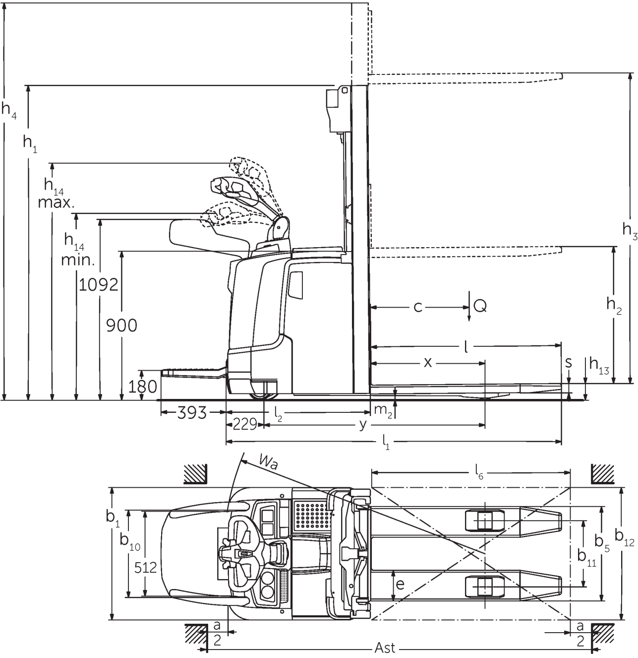
Maßzeichnung ERC 2
