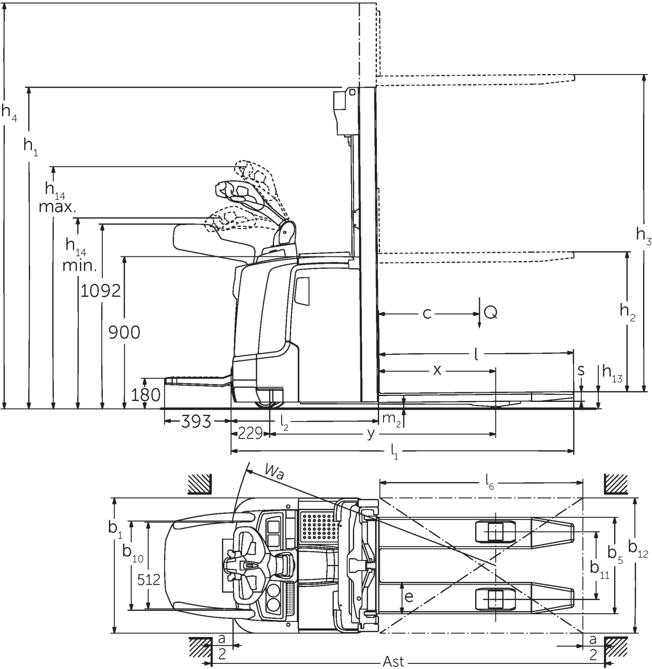
Méretezett rajz ERC 2
