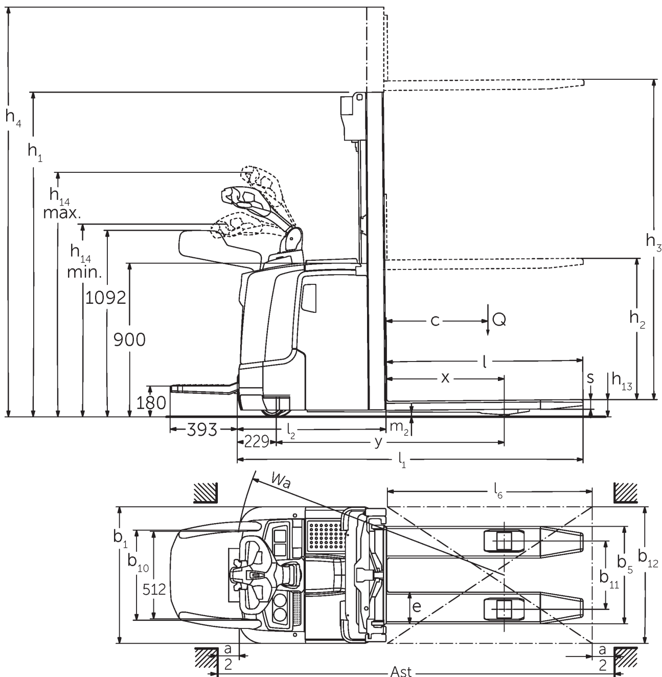
Výkres s rozměry ERC 2
