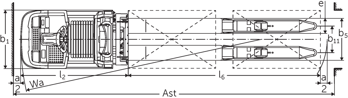
ECD 320 NOC 2016 tekn. tegn.
