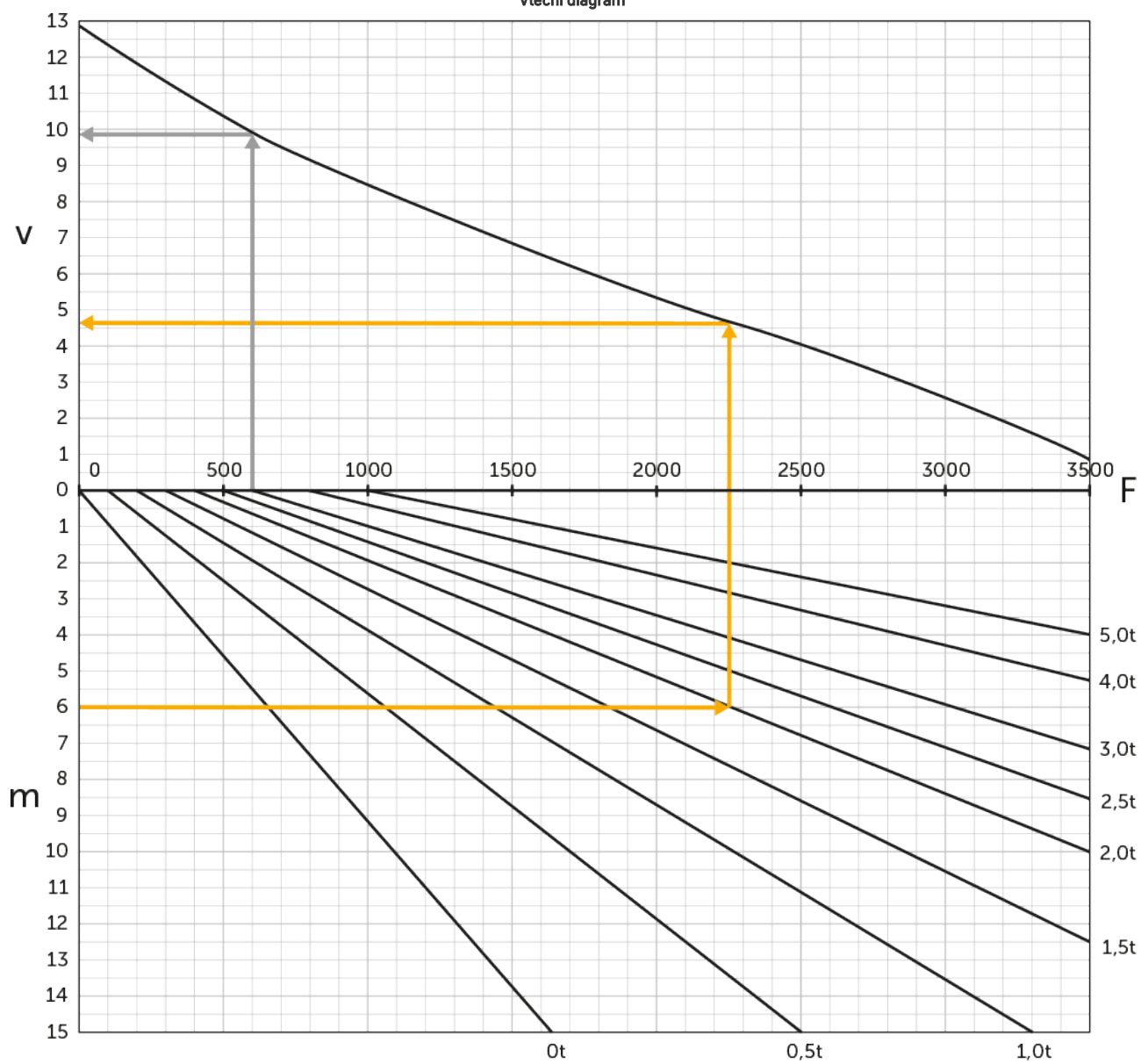
Vleční diagram
