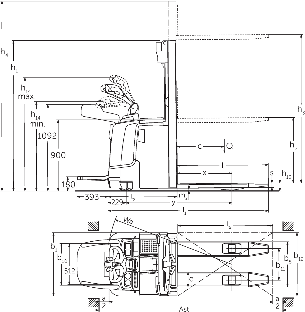
Tegning i målestokk ERC 2
