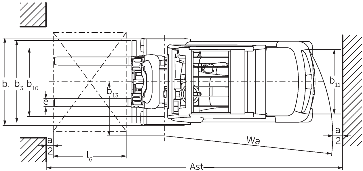
Dibujo técnico EFG 5 (2015)
