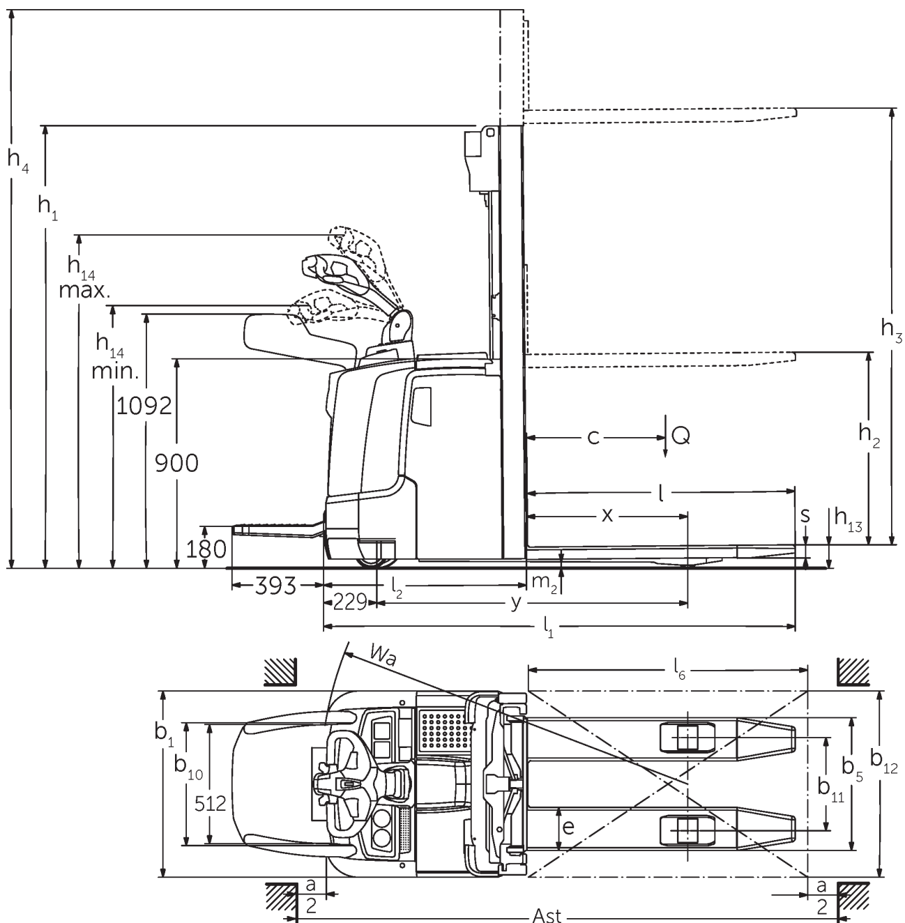
Mittapiirustus ERC 2
