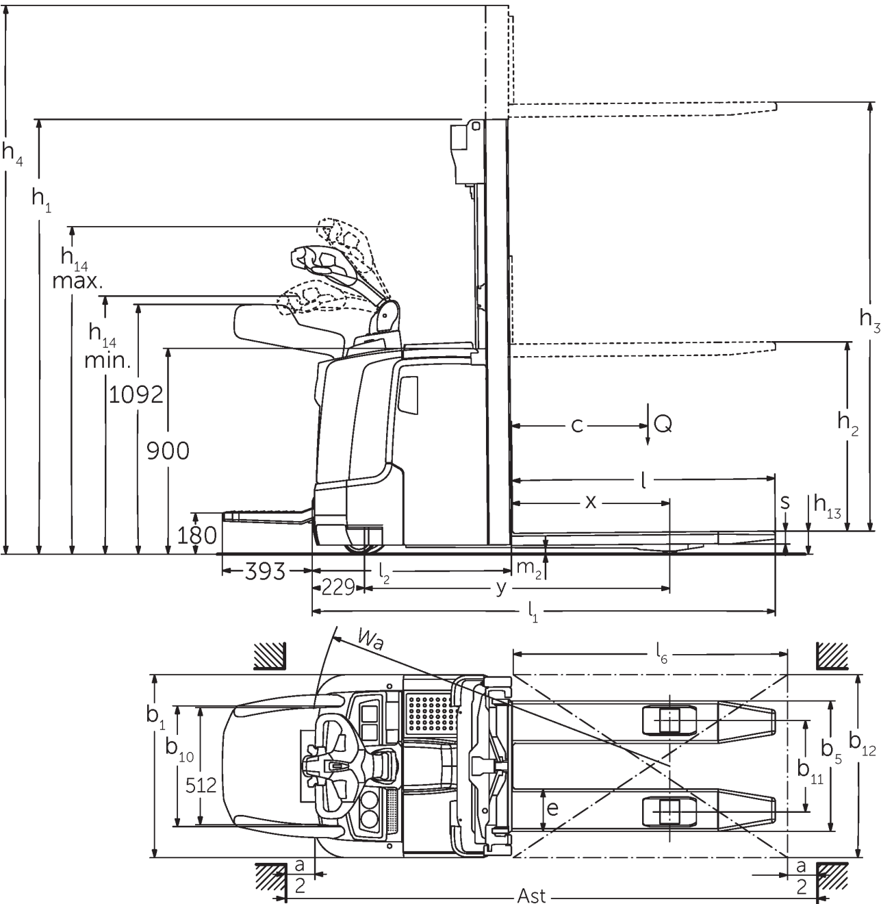
Mått ritning ERC 2
