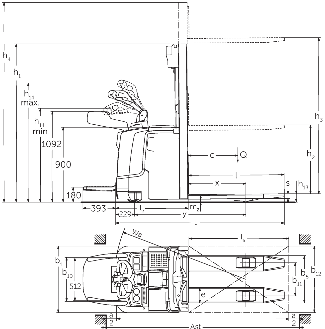
Mittapiirustus ERC 2
