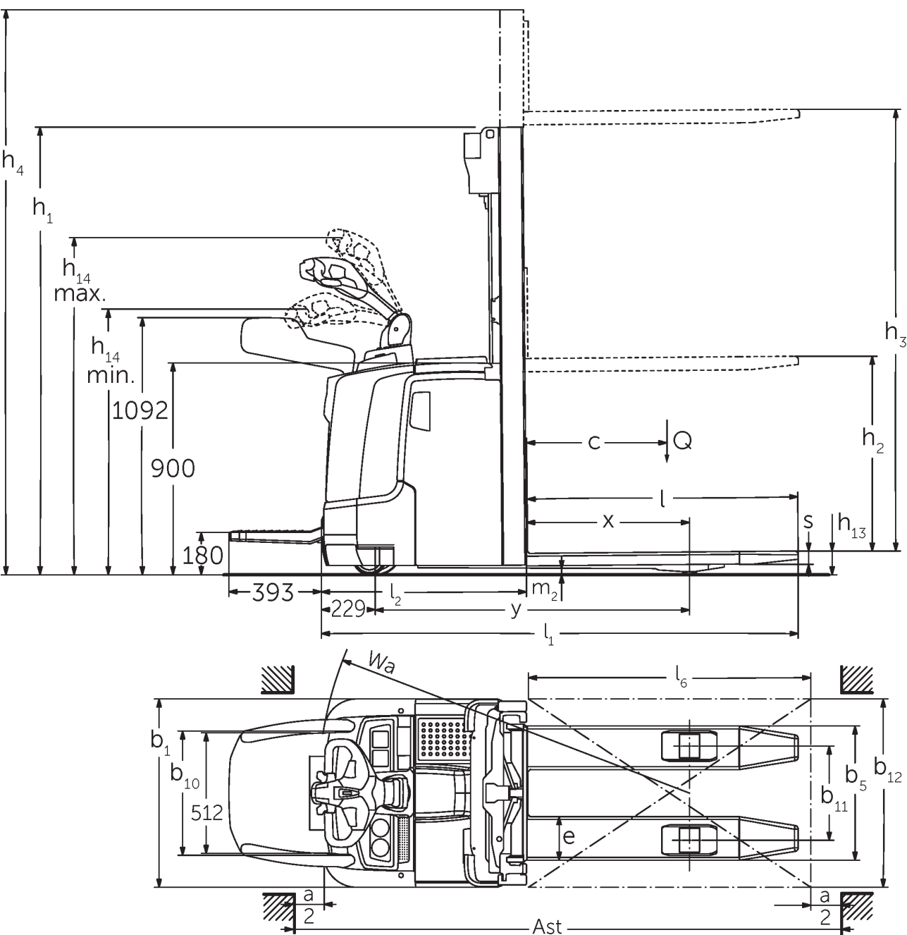
Måttavering ERC 2
