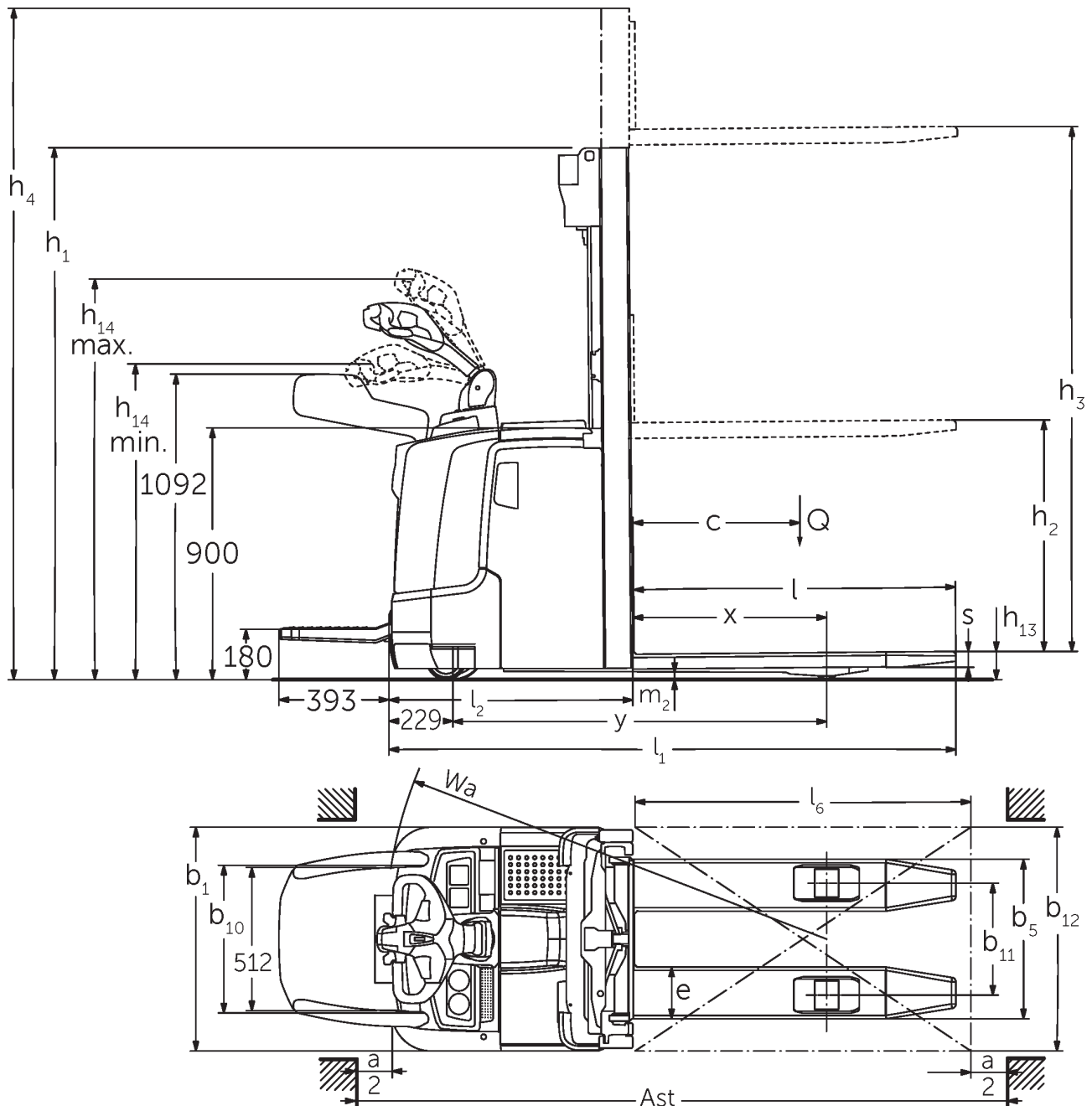
Maßzeichnung ERC 2
