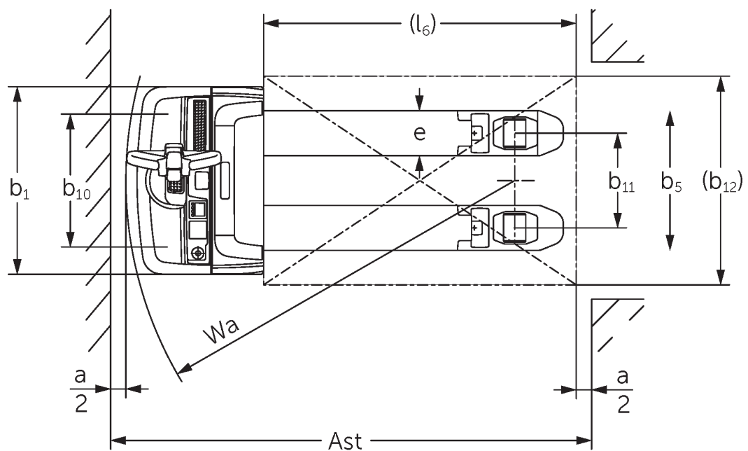
Viivapiirroksat EJE
