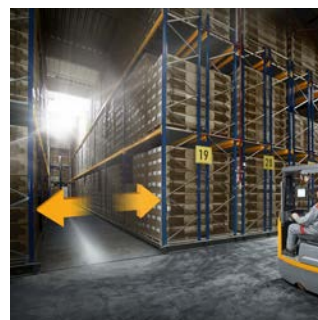
Večja učinkovitost: pri prevoznih regalih s povezavo WMS se hodnik odpre že ob približevanju.
