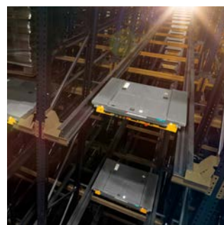
Jungheinrichov satelitski voziček UPC gre pod palete in ga je mogoče prilagoditi vašim potrebam.
