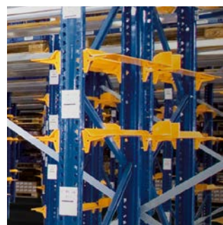
Enojni regal: kotni profili, razporejeni v smeri globine, prevzamejo funkcijo paletnega nosilca, kar omogoča dodaten prostor po višini.
