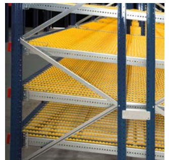
Individualna konfiguracija: pretočni regal za drobni material omogoča prilagodljivo nastavitve višine in kota nagiba.
